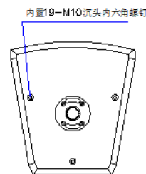
底视图/Bottom
