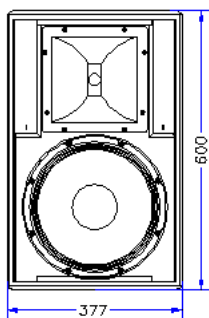
主视图/Front
