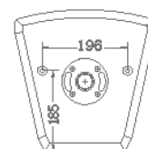
底视图/Bottom
